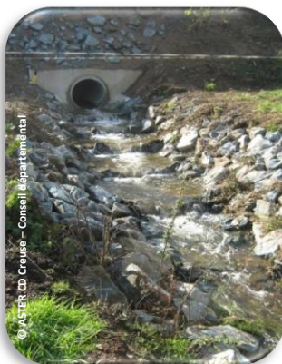
Passé à poissons de type rustique
